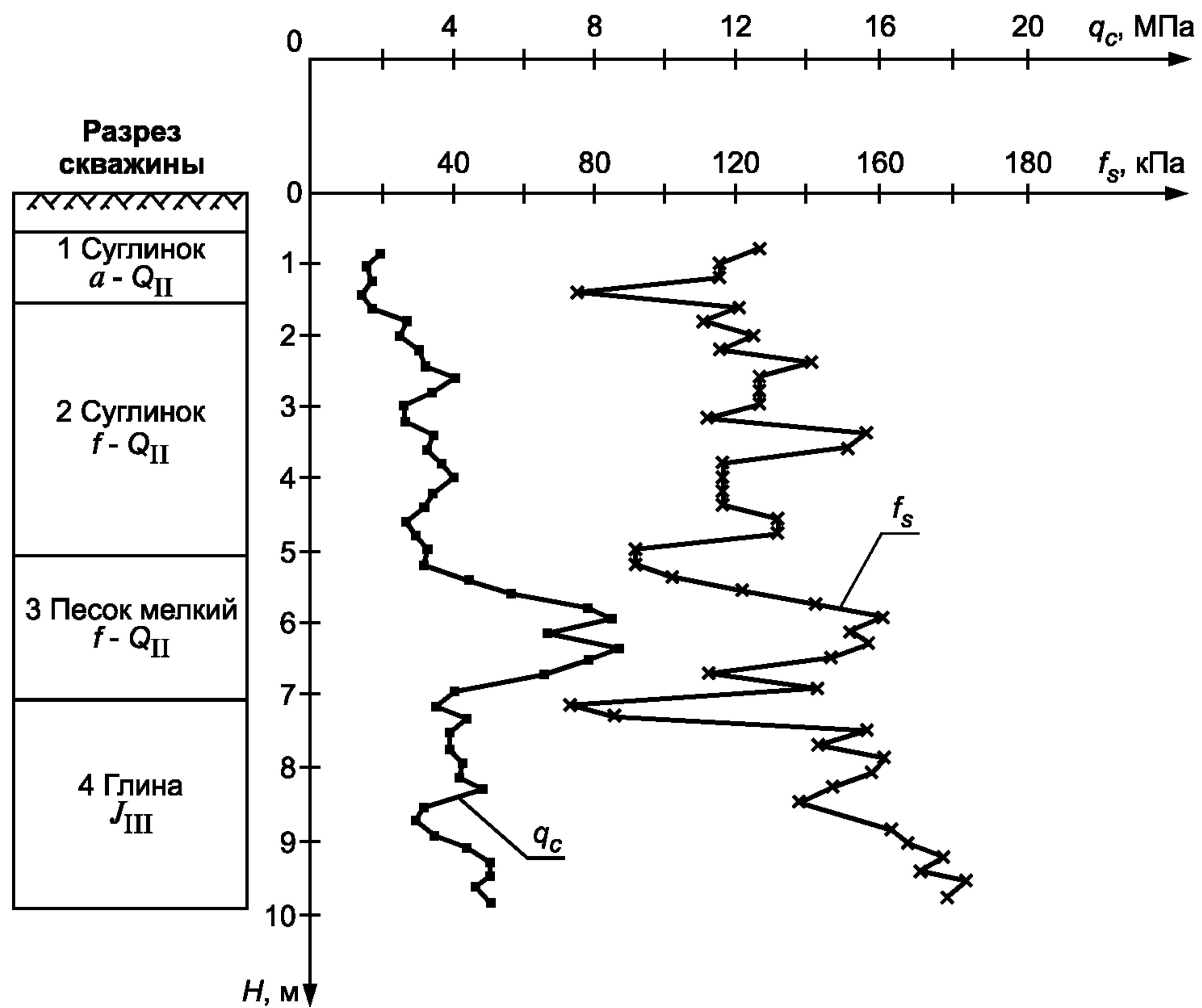
Рисунок В.2 — Графики изменения q_c и f_s в зависимости от глубины погружения зонда H
