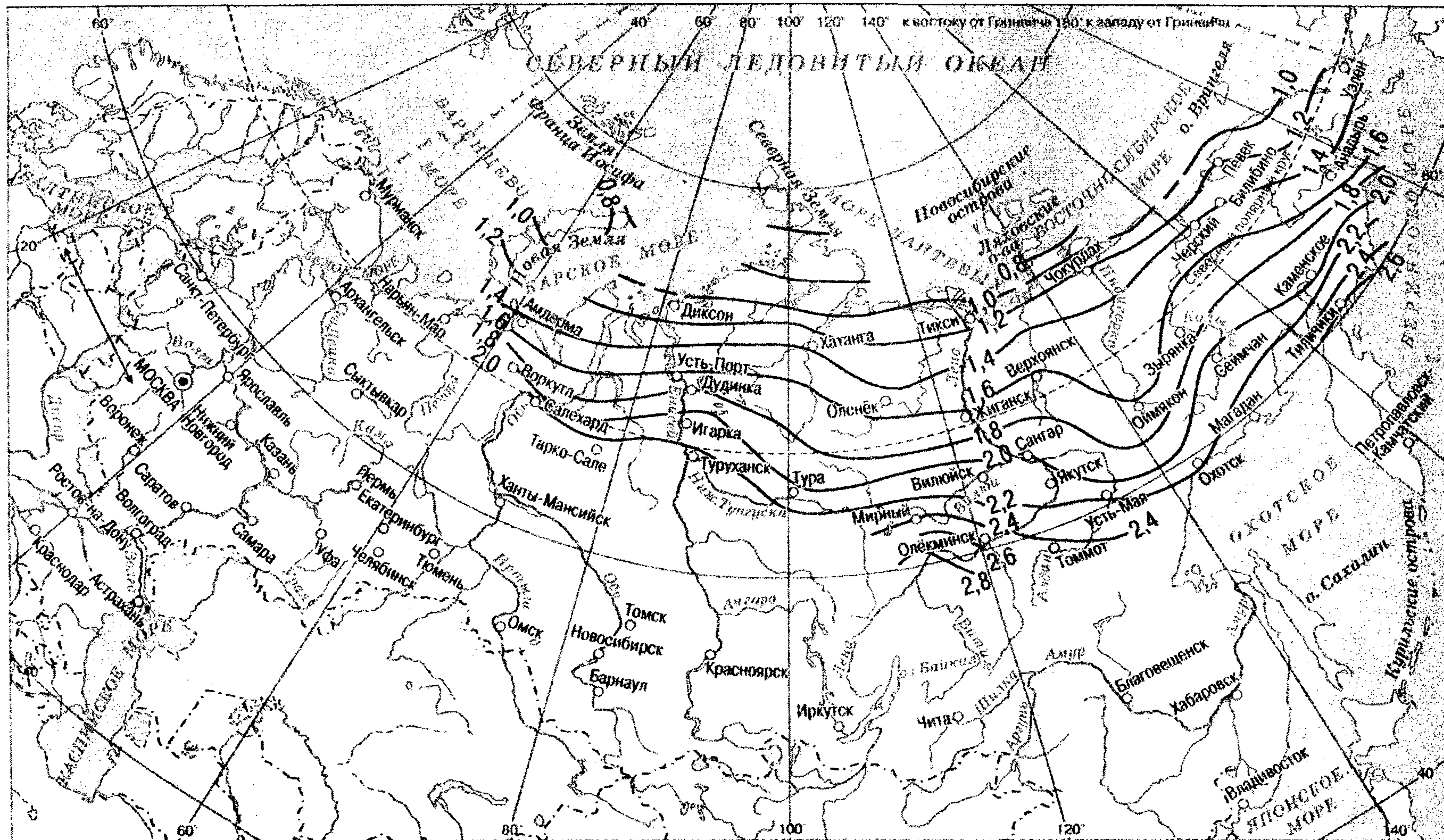
Рисунок Г.2 – Глубины оттаивания глинистых грунтов
