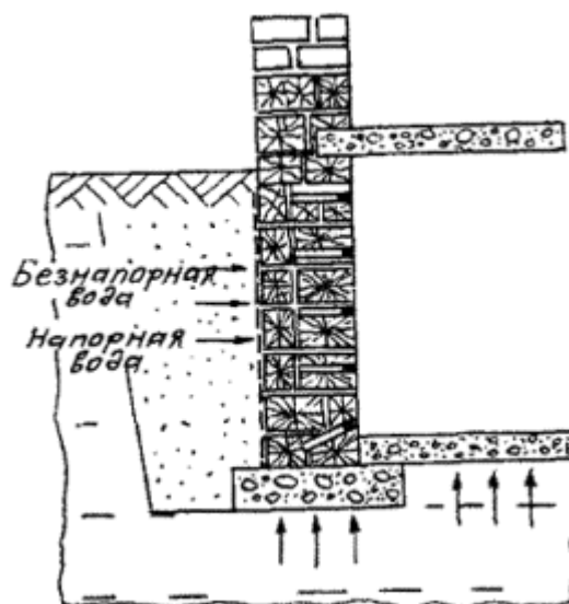
Рис. 3.8. Схема укрепления стен
