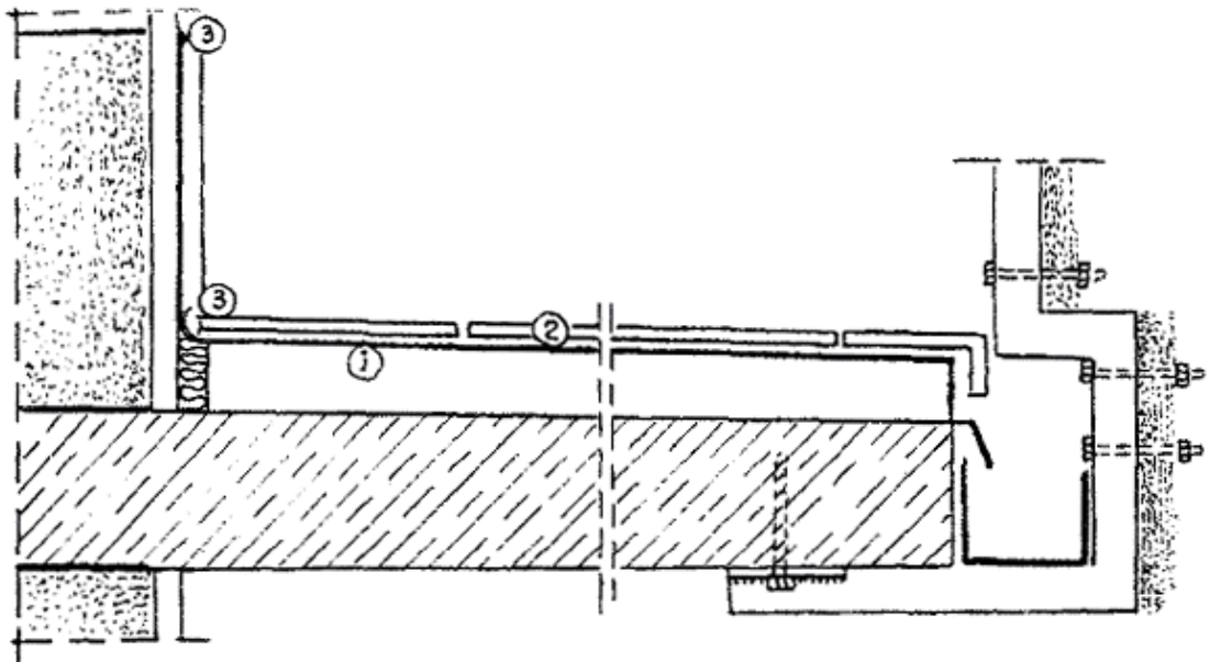
Рис. 4.9. Балконы и террасы. Гидроизоляция и ремонт:
