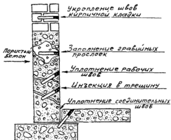
Рис. 3.5. Схема уплотнения отдельных негерметичных мест инъекции
