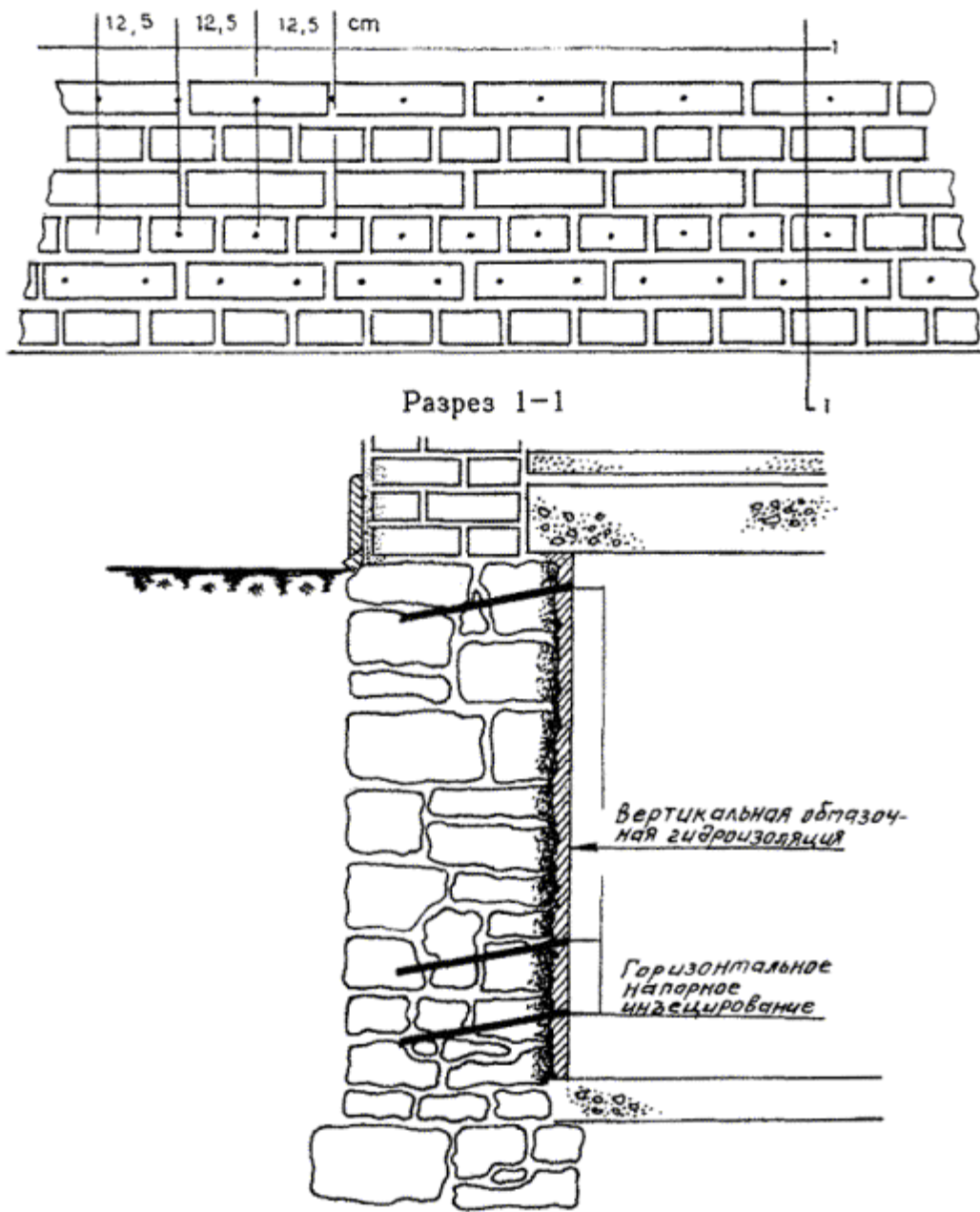
Рис. 3.3. Схема гидроизоляции подвала на объекте
