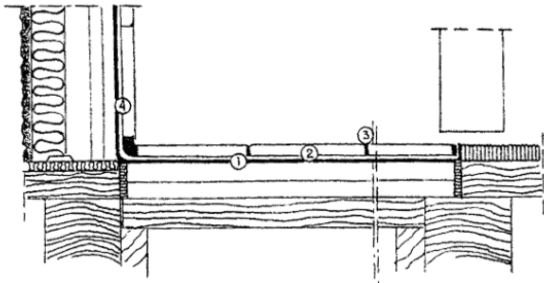
Рис. 4.4. Гидроизоляция под плитку. Постройки из легких конструкций (в частности, старые постройки):
