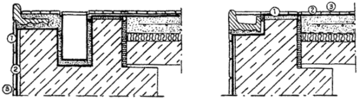
Рис. 4.5. Гидроизоляция плавательных бассейнов:
