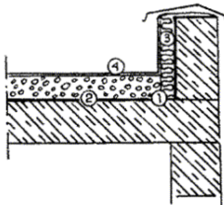
Рис. 4.7. Подземные гаражи:
