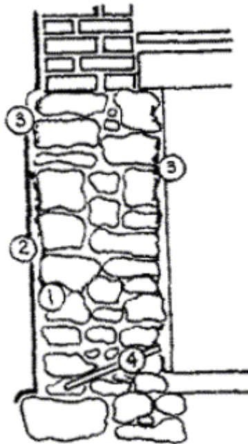
Рис. 4.8. Осушение каменной кладки преимущественно в старых постройках:
