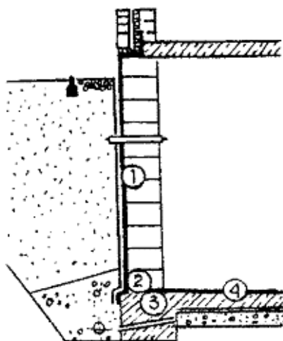
Рис. 4.1 Гидроизоляция подвалов и фундаментов в новостройках:
