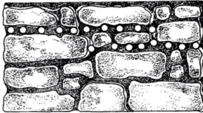
Рис. 3.1. Сверление отверстий в каменных конструкциях
