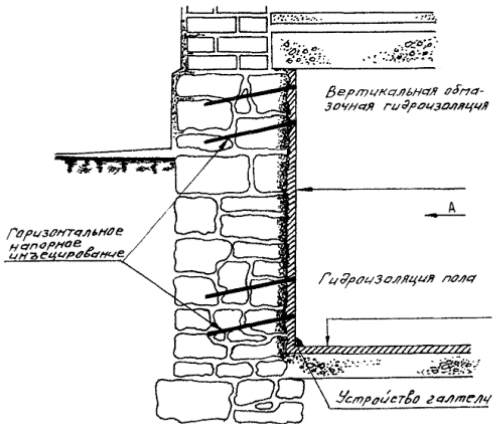
Рис. 3.4. Схема гидроизоляции подвала
