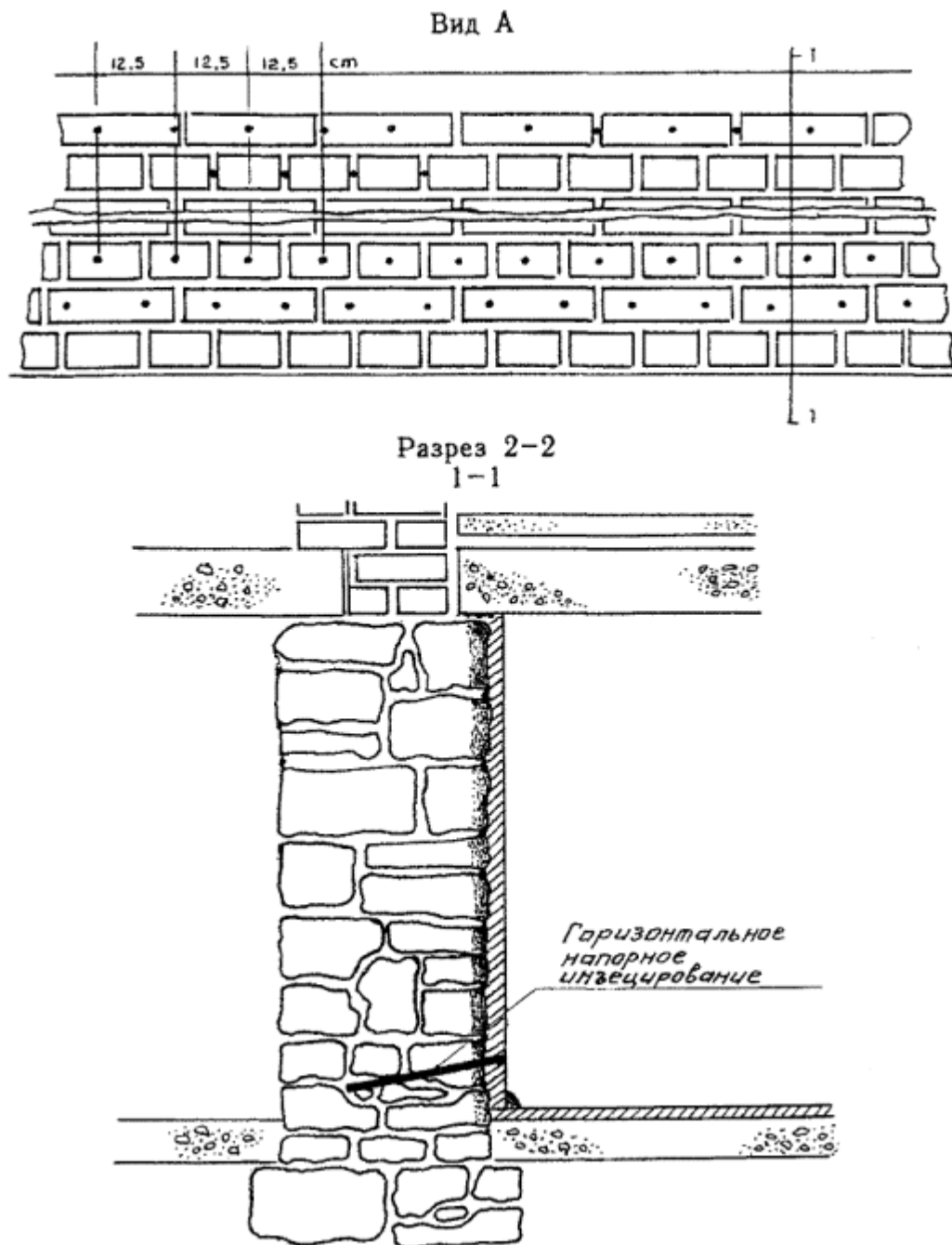
Рис. 3.2. Схема гидроизоляции подвала
