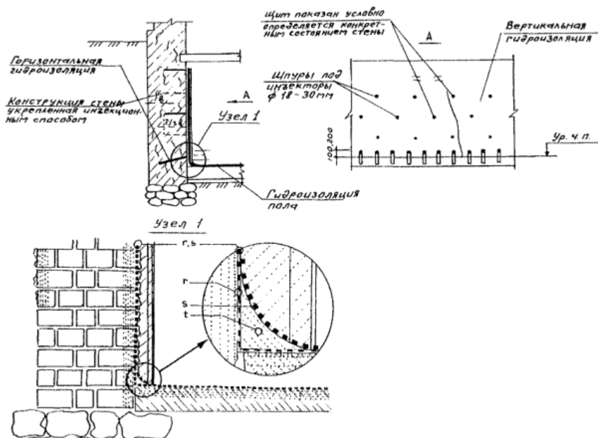
Рис. 3.7. Устройство инъекционной и покровной гидроизоляции
