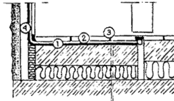
Рис. 4.3. Гидроизоляция под плитку. Капитальное строительство:
