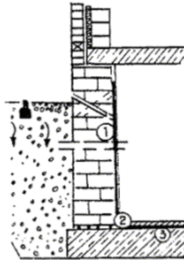
Рис. 4.2. Гидроизоляция подвалов изнутри в уже построенных зданиях:
